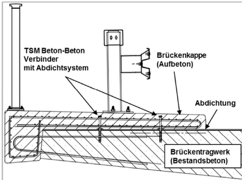
Verankerung mit einbetoniertem Verbinder
