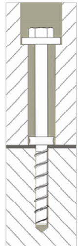
Verankerung mit nachträglich gesetztem Verbinder
