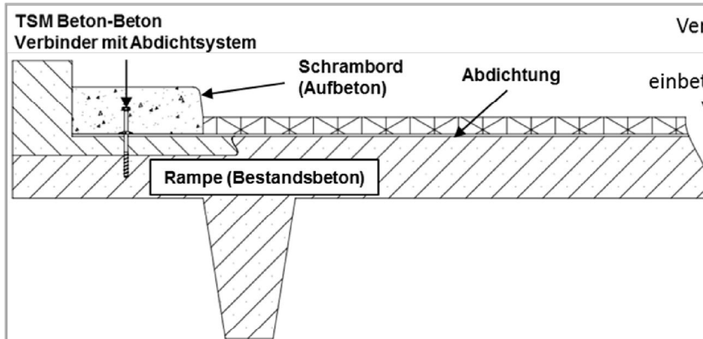
Verankerung mit nachträglich gesetztem Verbinder
