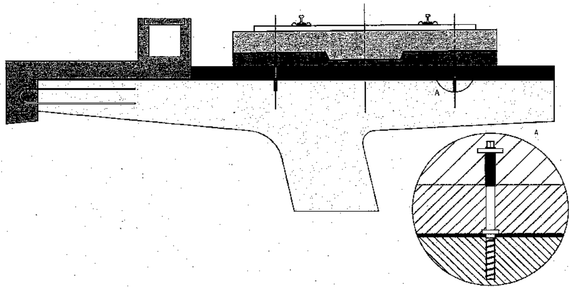
Abbildung 7: Befestigung der Höckerplatte durch einbetonieren der Verbundankerschrauben im Bereich der Höckerplatte
