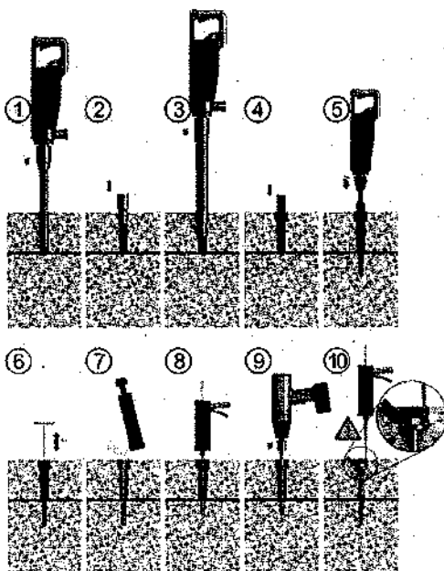
Abbildung 6: Verankerung von Brückenköpfen
